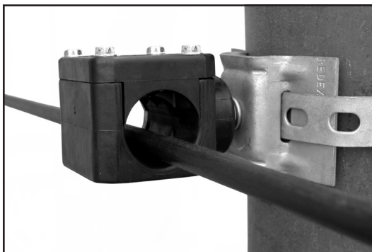
Foto 9 – Utilizando o FDS como dispositivo de lançamento.
