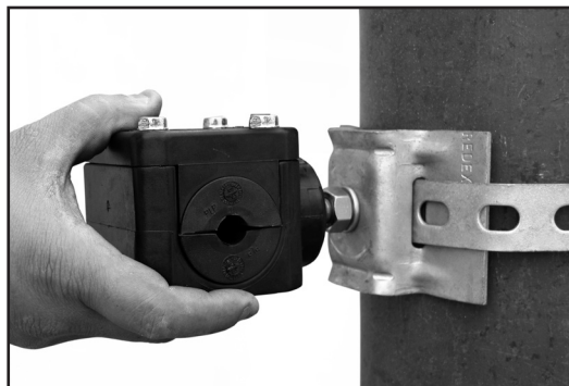
Foto 3 – Rosqueando o FDS.
