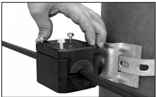
Foto 6 – Colocando a tampa no corpo do FDS.
