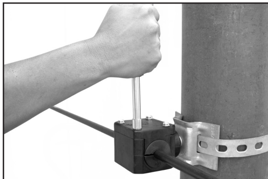
Foto 7 – Apertando os parafusos.
