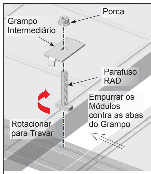
Figura 4: Instalando os Módulos utilizando Grampos Intermediários
