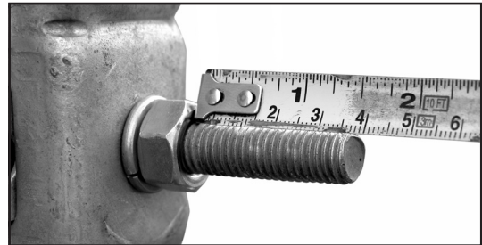
Foto 2 – Medindo o comprimento da Rosca.
