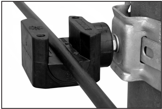
Foto 4 – Colocando o cabo no berço do coxim.
