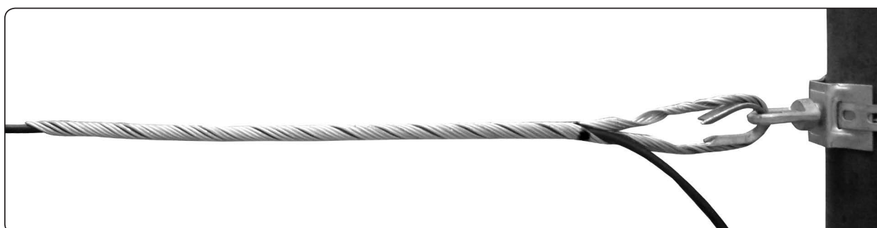
Alça Preformada aplicada com Kit BAP
